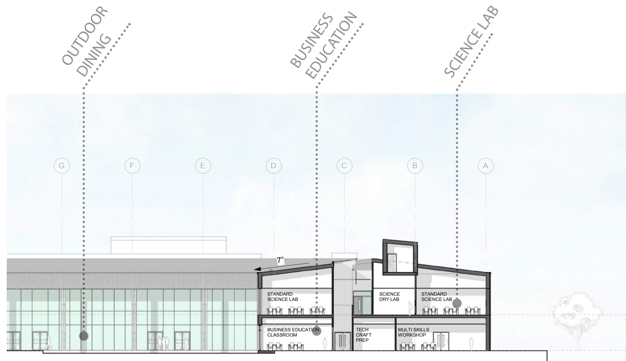
SECTION A-A
