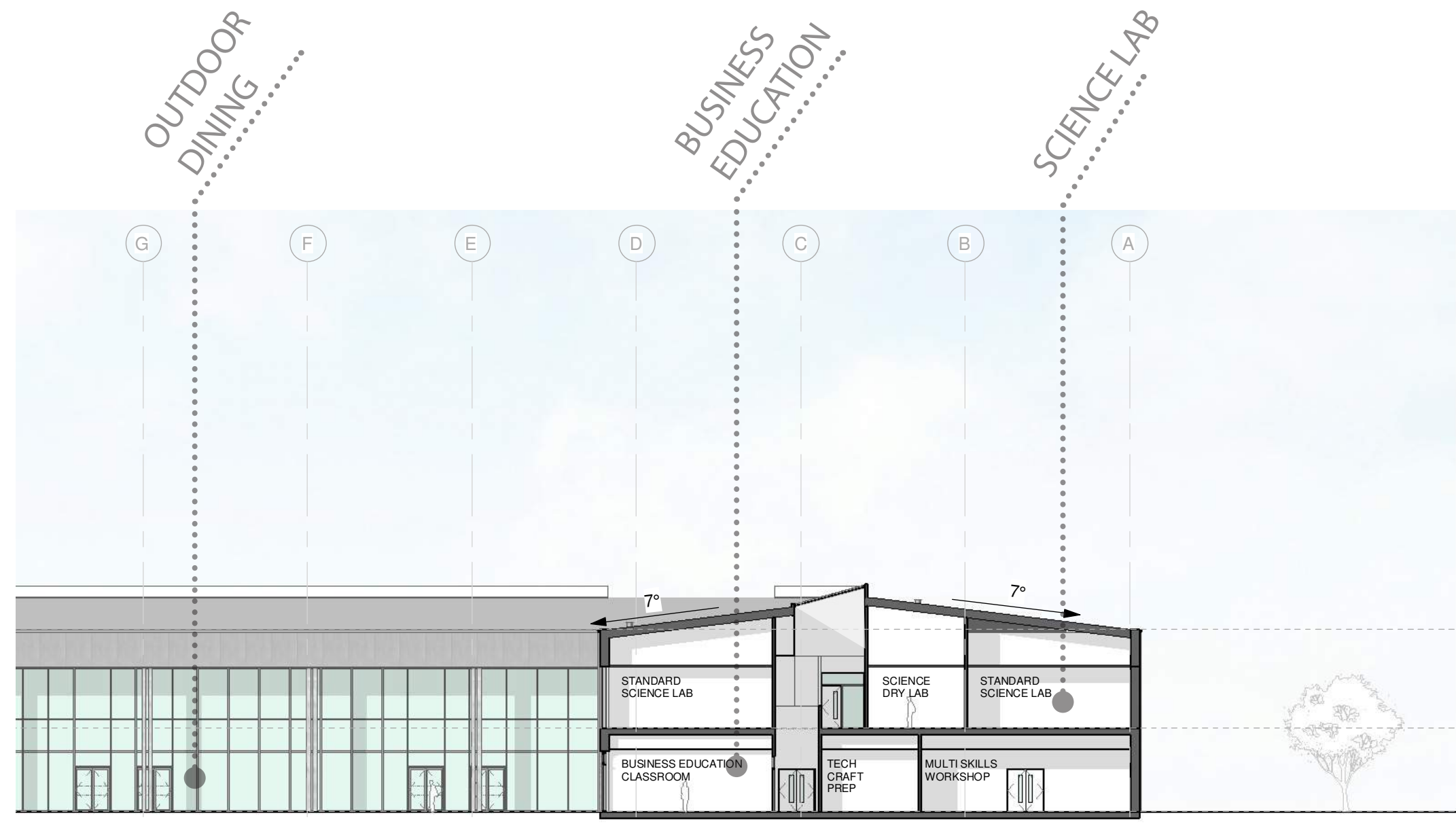
SECTION A-A
