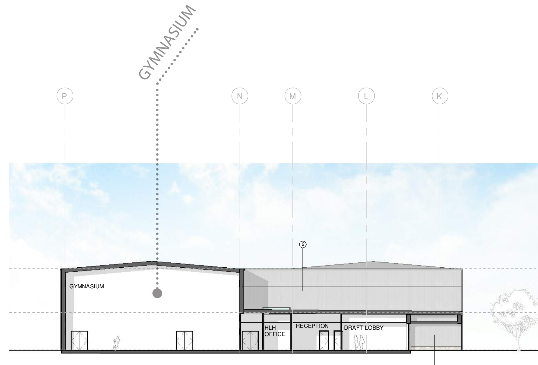
SECTION D-D
