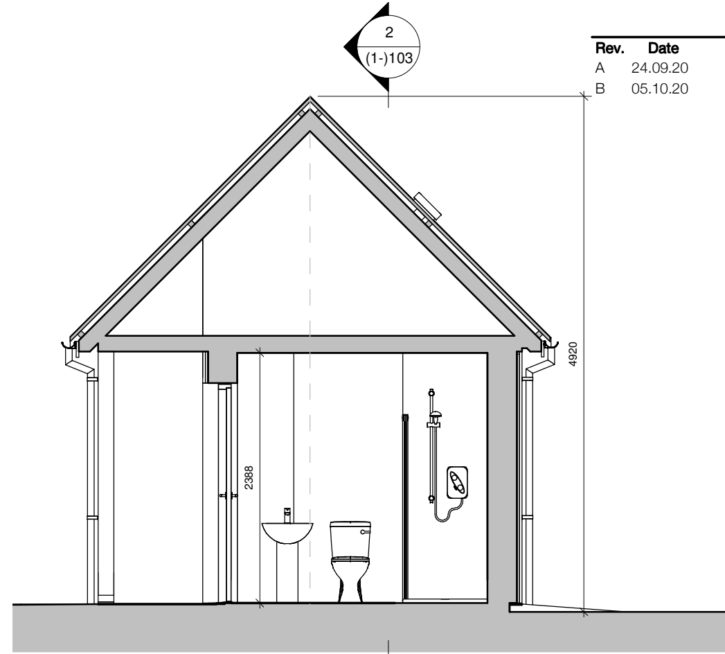
3 Section 2 1 : 50
