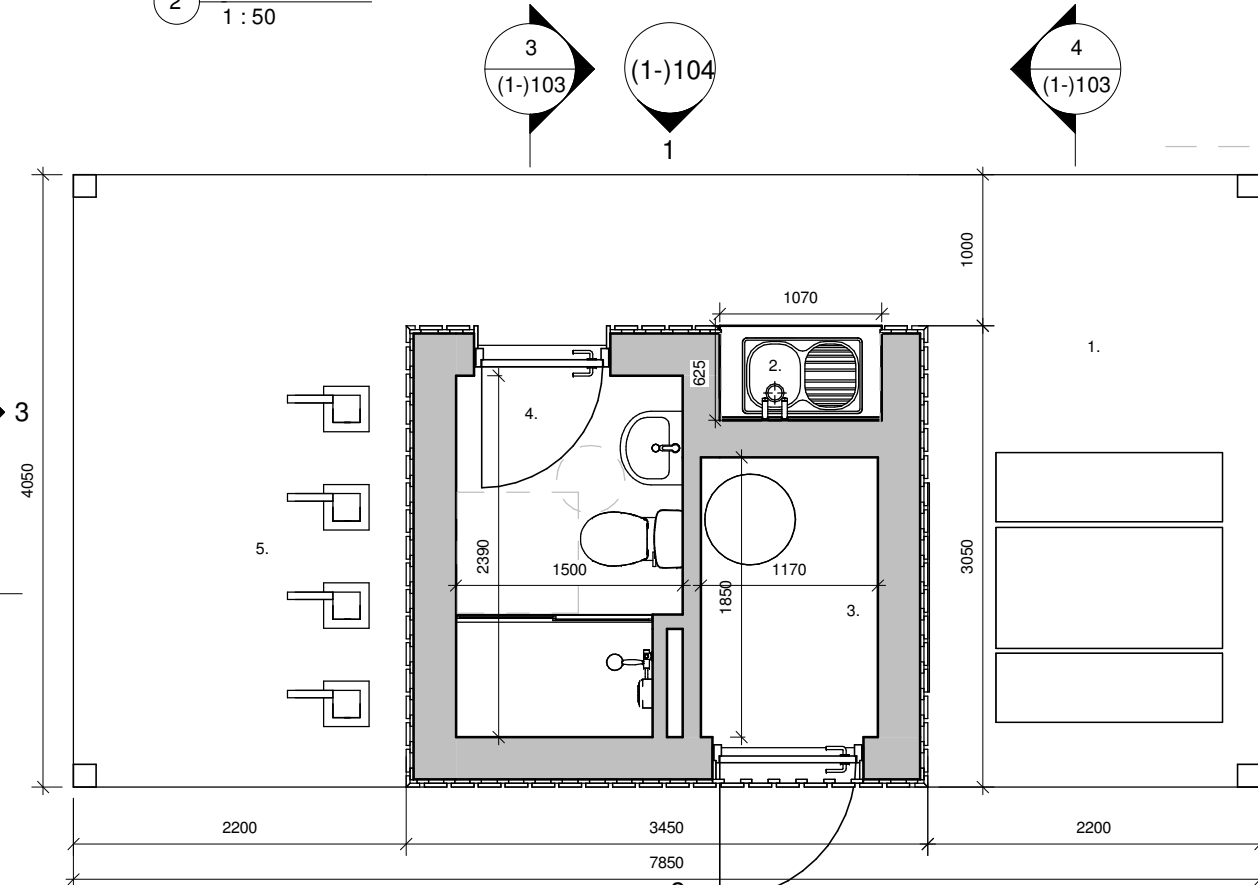
1 Floor Plan 1 : 50
