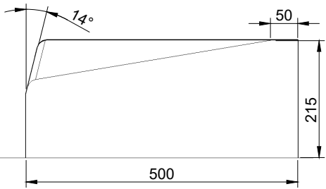
End Elevation (LH unit)
