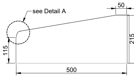
End Elevation
