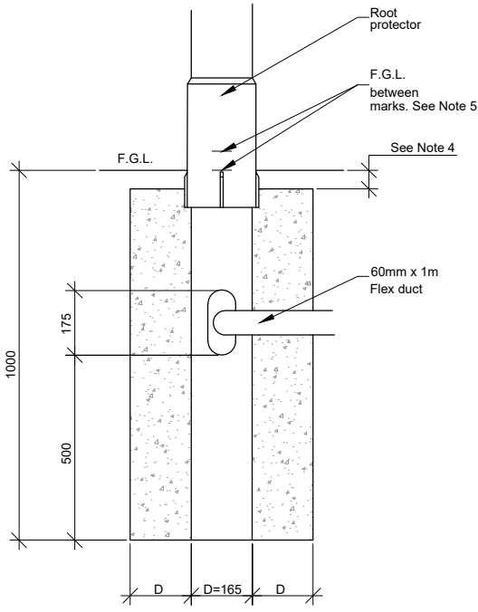
6m column
